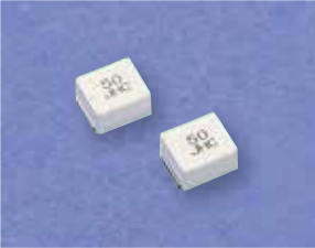
JHC型 Nシリーズ7358(30A~100A) Type JHC N Series 7358(30A~100A) (L:7.3×W:5.8×T:4.2mm) 250%溶断品 250% of rated current AEC-Q200準拠品
