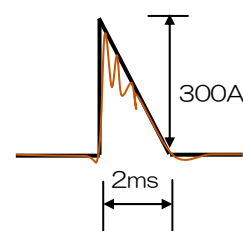
図C：突入電流波形（模式図）
