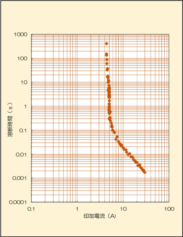
JAE 2402 252NA52010 n=100 個
