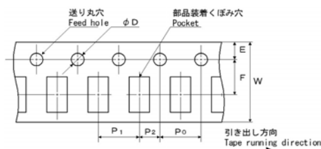
テーピング寸法/Tape dimensions
