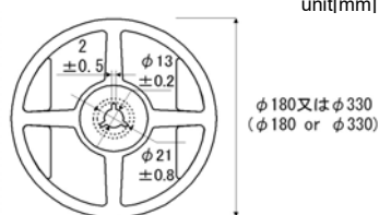
リール寸法/Reel dimensions
