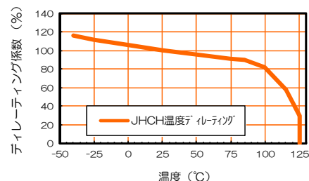
図B：温度ディレーティング
