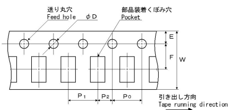
テーピング寸法/Tape dimensions
