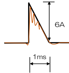
図C：突入電流波形（模式図） 赤線：実測波形 黒線：近似波形
