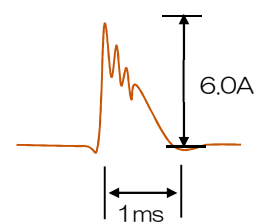
図A：突入電流波形
