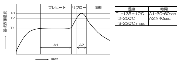
図1 [10V470μF (Hケース)のIRリフロー法]
