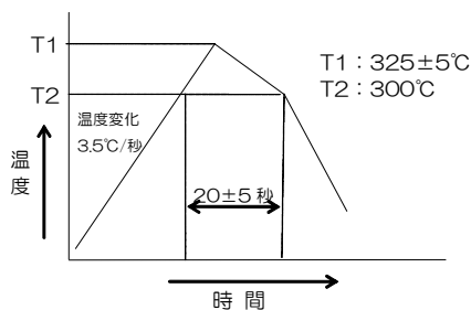
図1 I Rリフロー温度プロファイル
