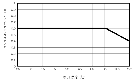
図1 電圧軽減曲線（推奨）
