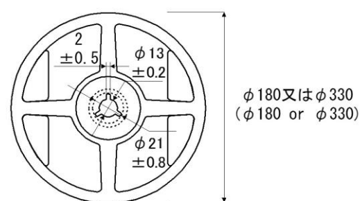
リール寸法/Reel dimensions
