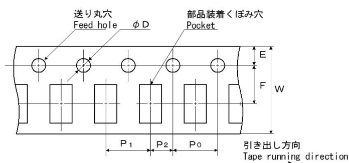
テーピング寸法/Tape dimensions
